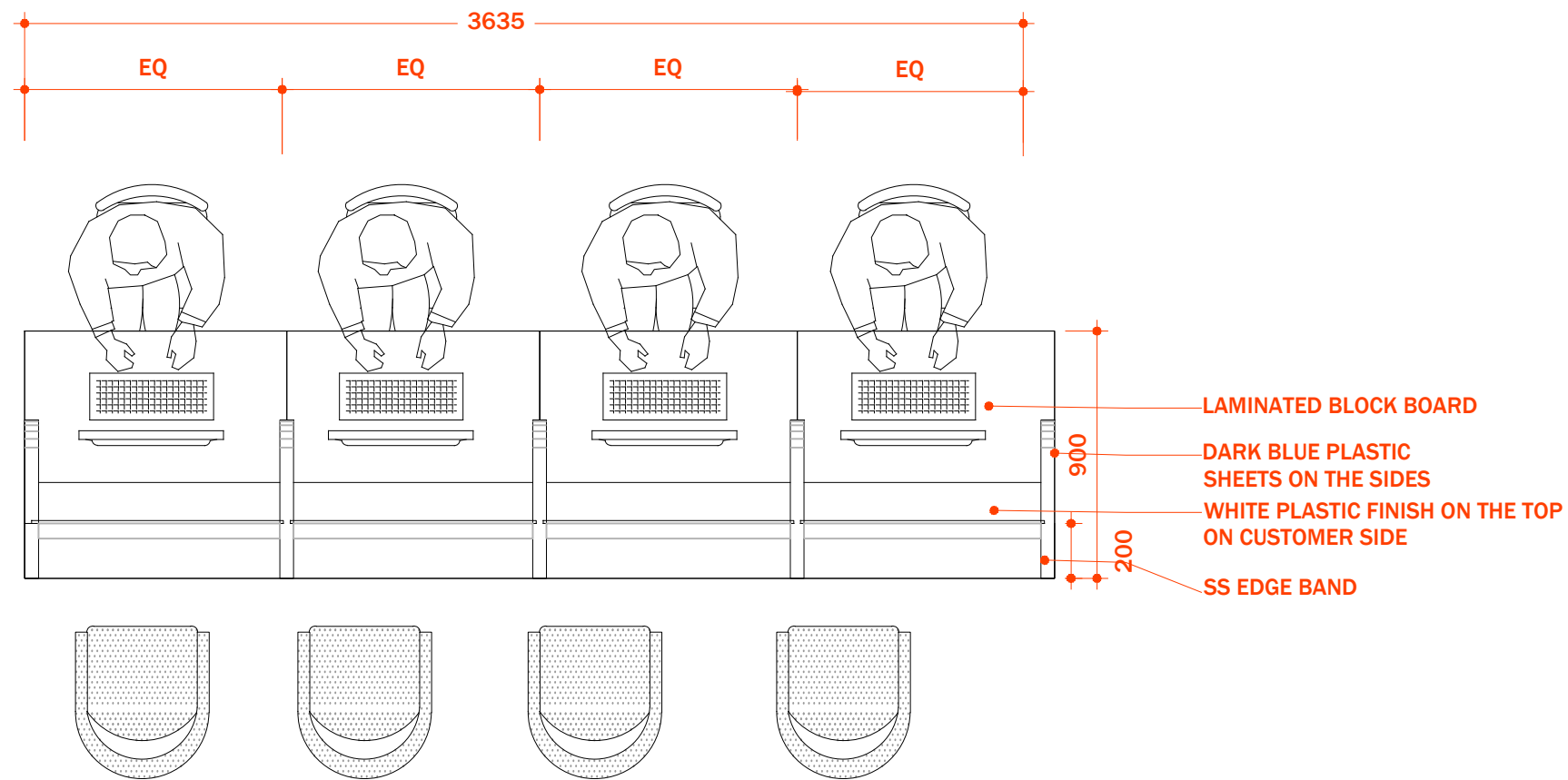
1 PLAN VIEW SCALE: 1:50
