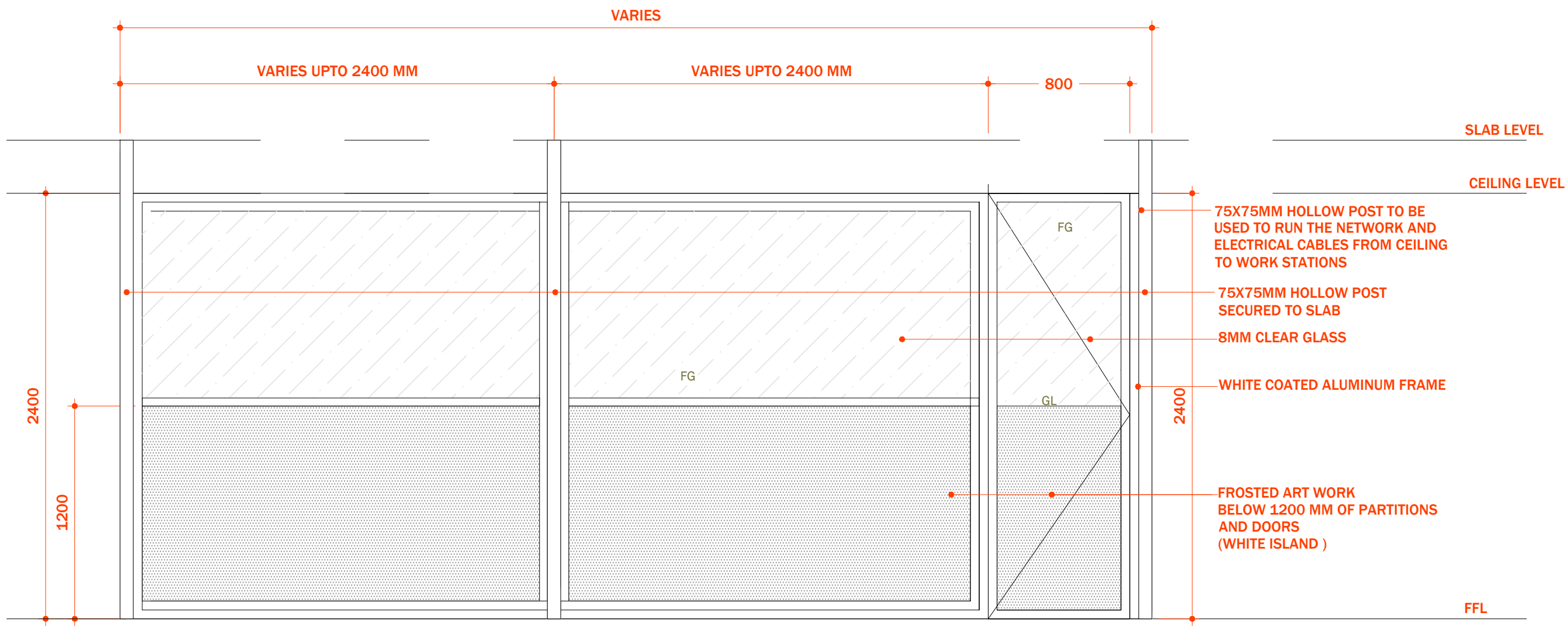
1 PARTITION DETAIL 01 SCALE: 1:50
